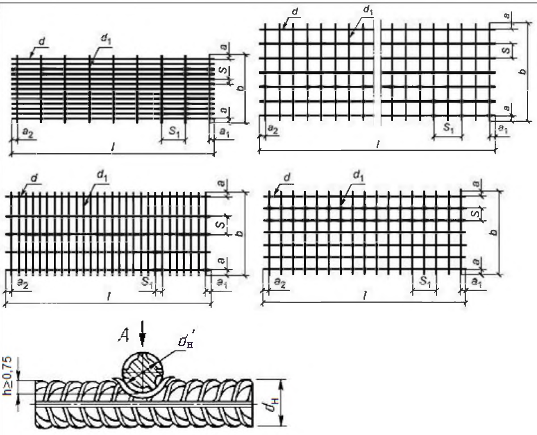
Крестообразное соединение арматуры
